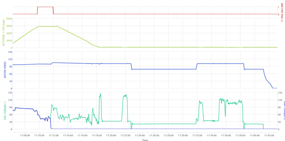
Plottaggi di dati estratti da FDR ed elaborati per l'analisi.
