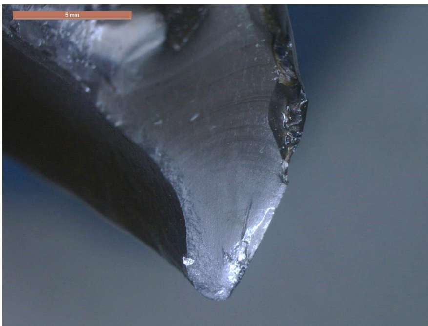
Superficie di rottura di un componente investigato dai laboratori della ANSV, caratterizzato da una rottura per fatica.
