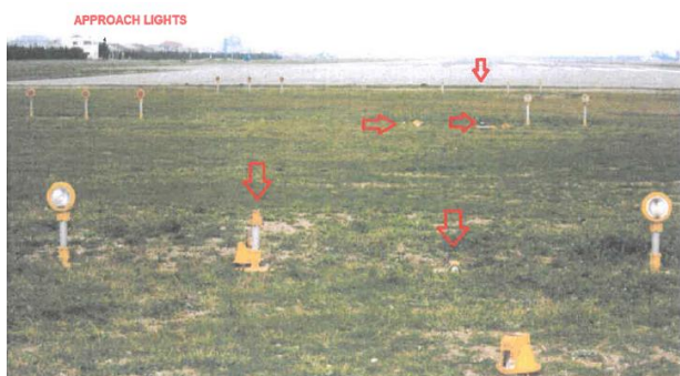
Foto dei danni alle luci del sistema luminoso di avvicinamento e all'antenna del localizer .
