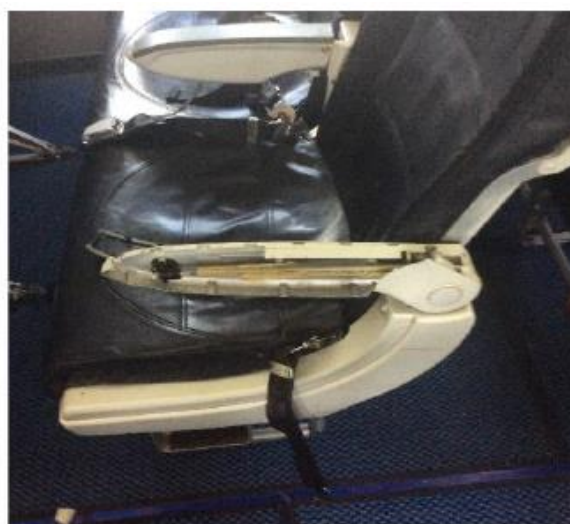
Particolare dei danni causati dall'urto dell'assistente di volo feritosi nell'evento (foto effettuate dall'operatore).
