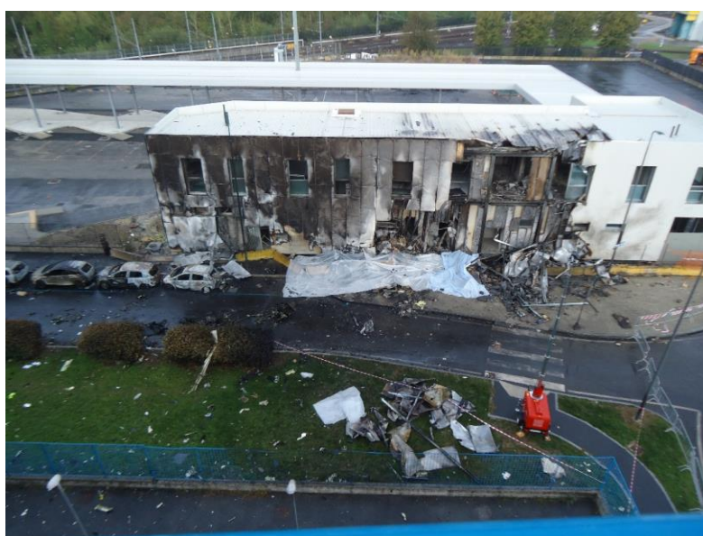
Luogo dell'incidente e resti del velivolo Pilatus PC-12 marche YR-PDV.
